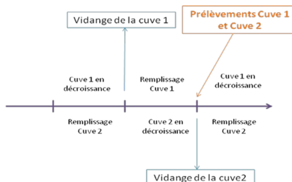
Figure 2 : Principe de gestion des deux cuves de décroissance du GIP CYCERON
