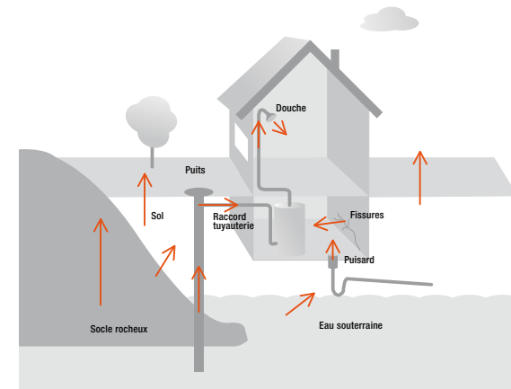
Infiltration du radon dans une maison
